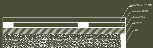
SEC D-D
